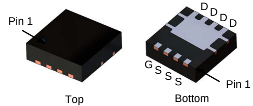
PQFN8 3.3X3.3, 0.65P (Power 33) CASE 483AK
