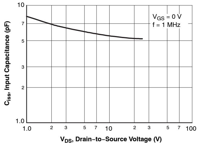
Figure 8. C_{iss} - V_{DS}
