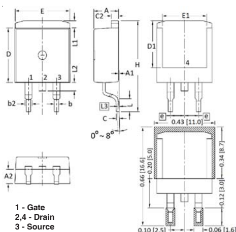
TO-263 Outline
