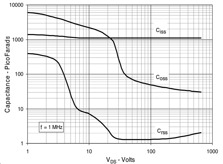
Fig. 12. Capacitance
