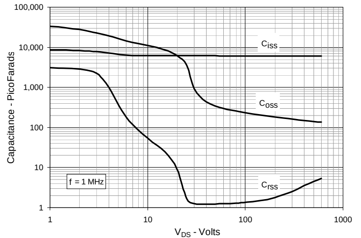
Fig. 12. Capacitance
