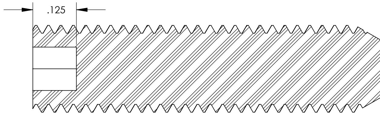
SECTION A-A
