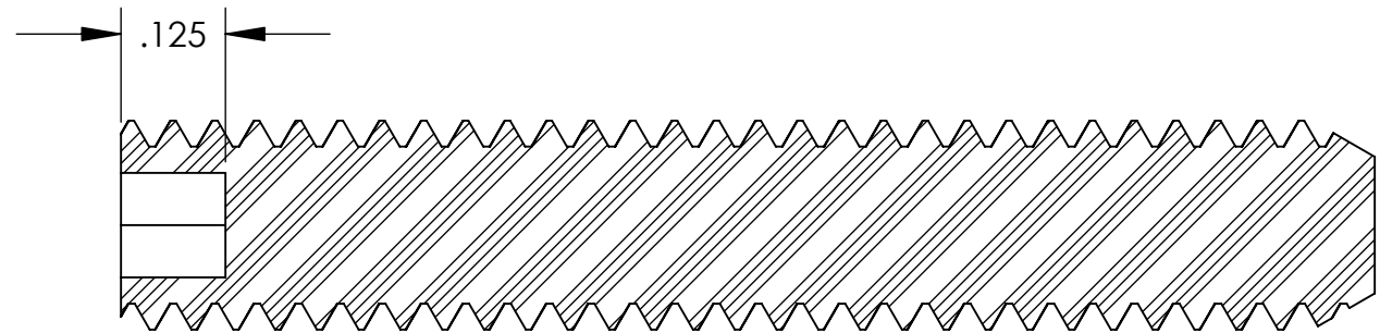
SECTION A-A
