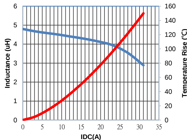
MGV12054R7M-10
