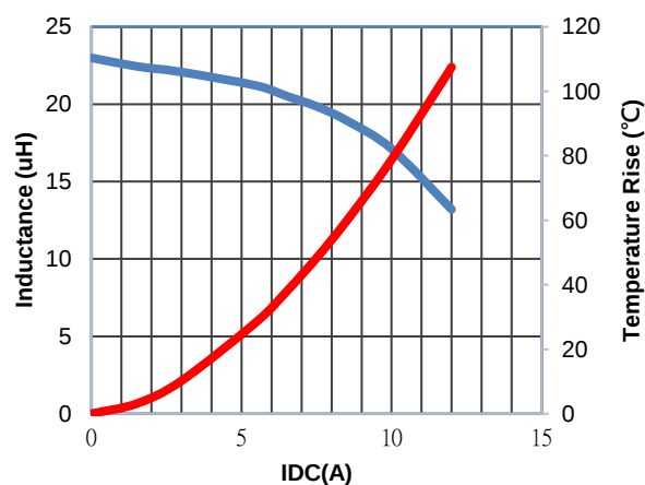
MGV1205220M-10
