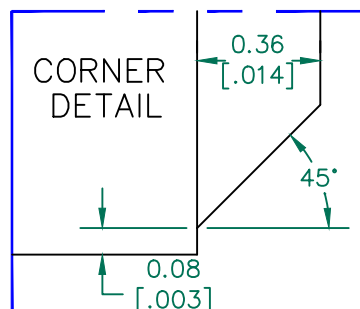
DETAIL "A" SCALE: 50 : 1
