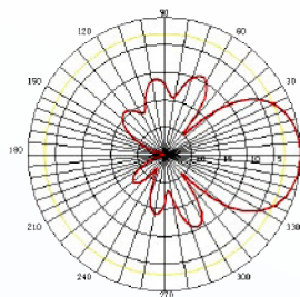
YA9-11 H-Plane
