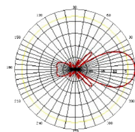
YA9-13 E-Plane
