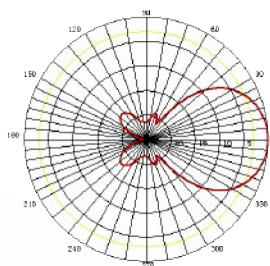
YA9-11 E-Plane
