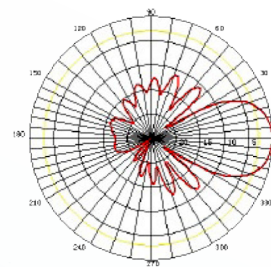
YA9-13 H-Plane
