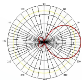
YA9-9 E-Plane
