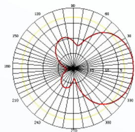
YA9-9 H-Plane
