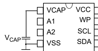
Fig. 10: PowerStore Configuration
