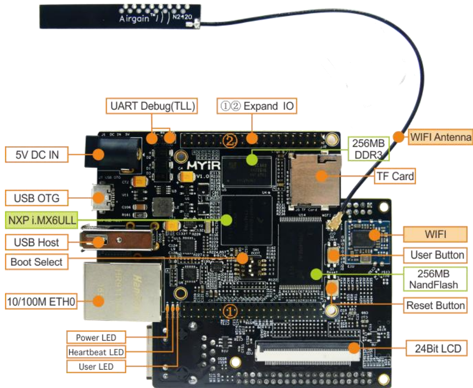
MYS-6ULX-IOT
