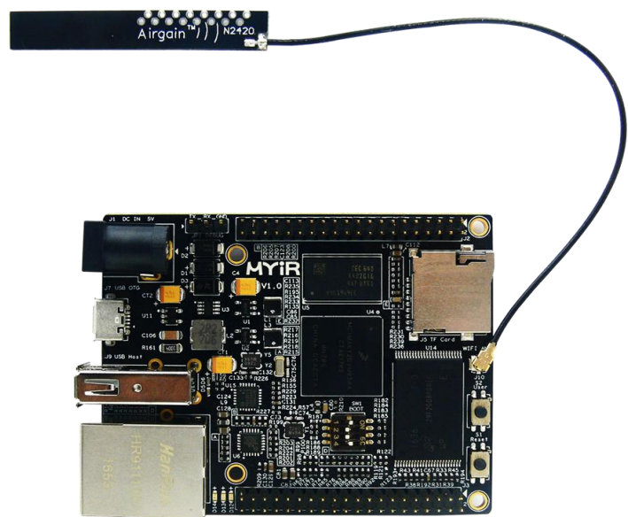
MYS-6ULX-IOT
