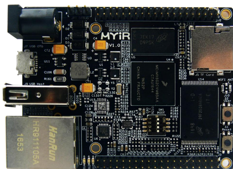
MYS-6ULX-IND
