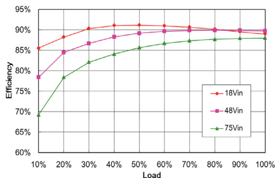
QSB40048S28
