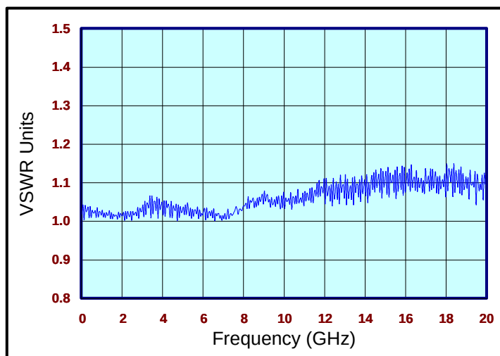
PN: CCSMA-MM-SS402-120 VSWR (S22)
