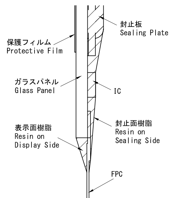
B部拡大図 (10 : 1)
