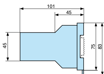
26546840 - DIN rail adaptor
