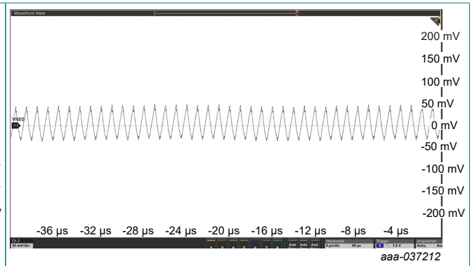
Fig. 31. V_{NEG} output ripple ( I_{NEG} = 220 mA)
