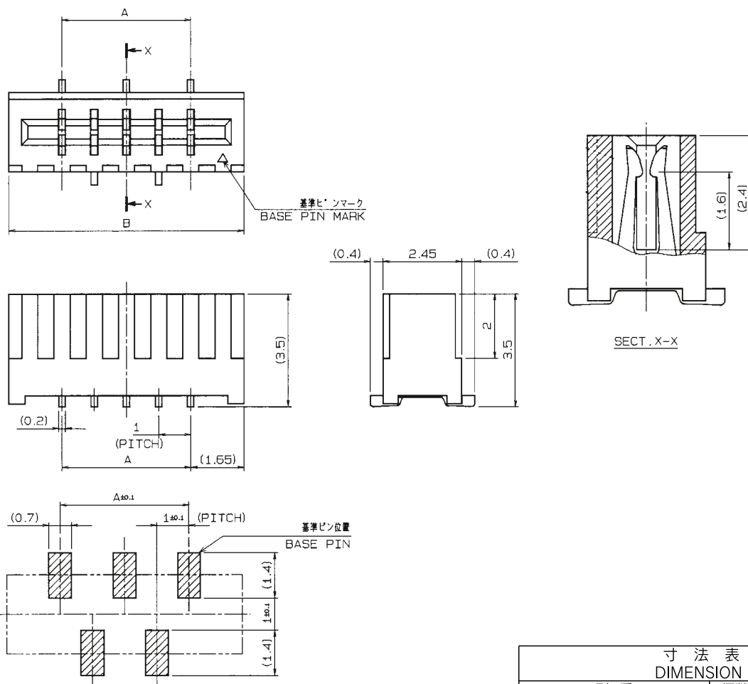
基板取付け寸法 (コネクタ搭載面側) MOUNTING LAYOUT (CONN. MOUNTING SIDE)
