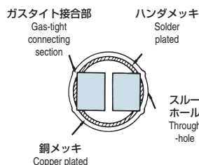
断面 Cross section
