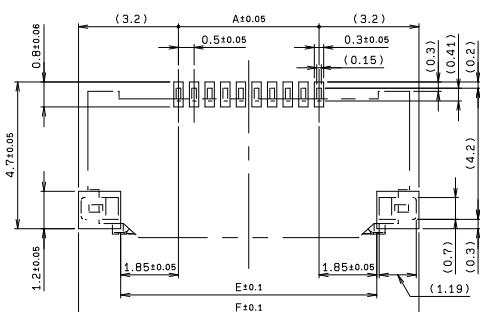
推奨パターン寸法 RECOMMENDED PATTERN LAYOUT
