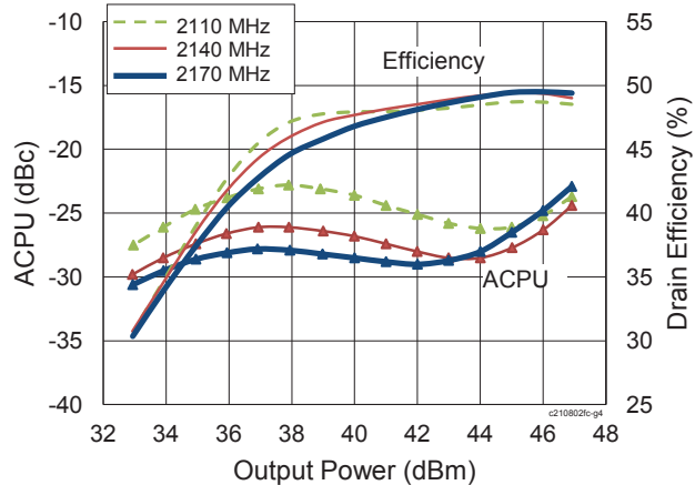
Single-carrier WCDMA Drive-up V_{DD} = 28\text{ V} , I_{DQ} = 100\text{ mA} , V_{GS1} = 1.3\text{ V} , 3GPP WCDMA signal, PAR = 10 dB, BW 3.84 MHz
