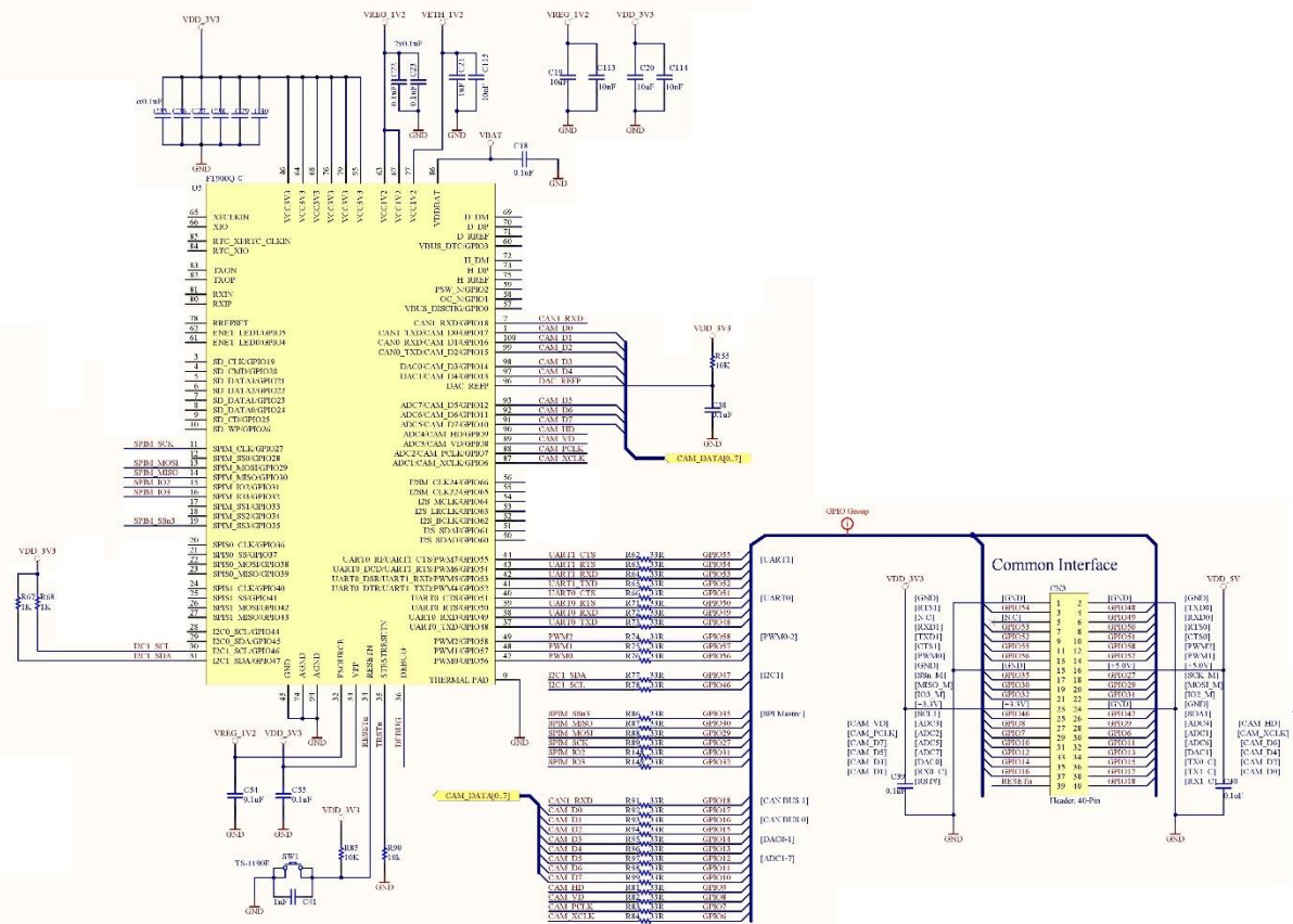
FT900 Module
