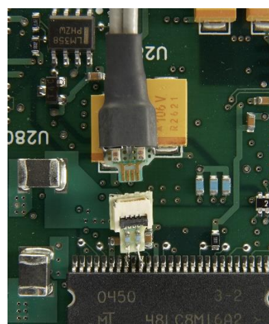
Figure 10: N5425B/26A differential ZIF head and ZIF tip
