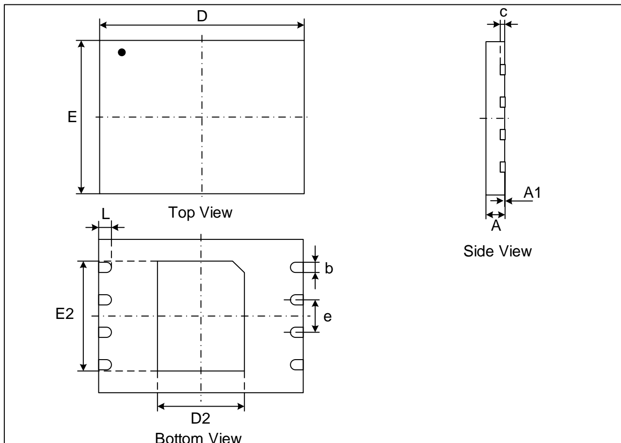
Figure21-1. WSON8 (6*8mm)
