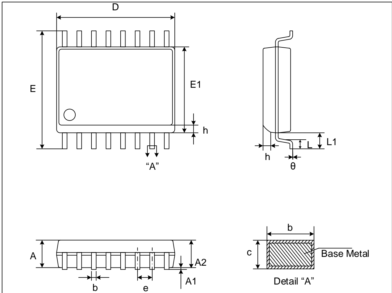
Figure21-2. SOP16 300MIL
