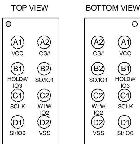
WLCSP
