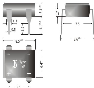
Dimensions - Maße [mm]
