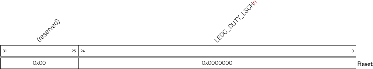
Register 14.8. LEDC_LSCH n _DUTY_REG ( n : 0-7) (0xA8+0x14* n )
