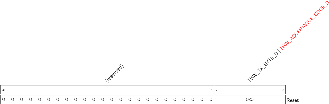
Register 21.5. TWAI_DATA_O_REG (0x0040)
