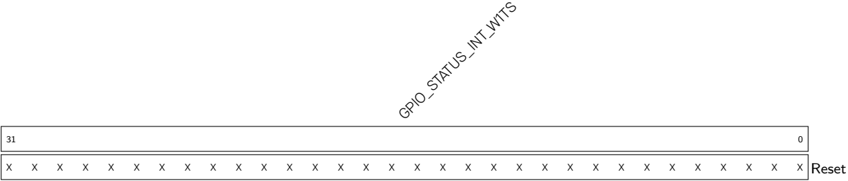
Register 4.17. GPIO_STATUS_W1TS_REG (0x0048)
