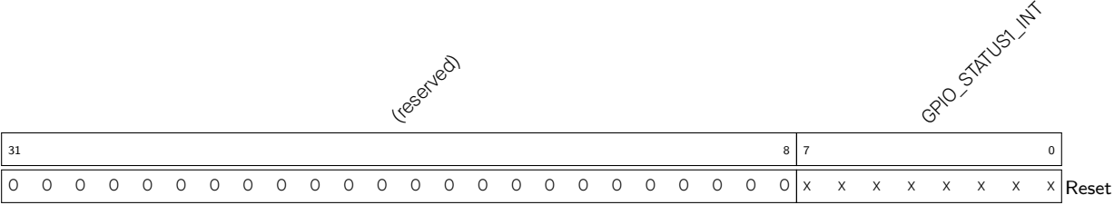
Register 4.19. GPIO_STATUS1_REG (0x0050)
