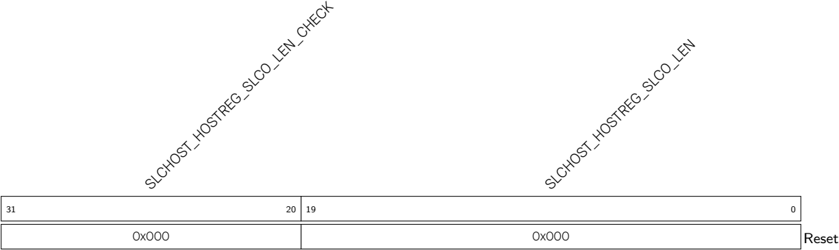
Register 8.17. SLCHOST_PKT_LEN_REG (0x60)
