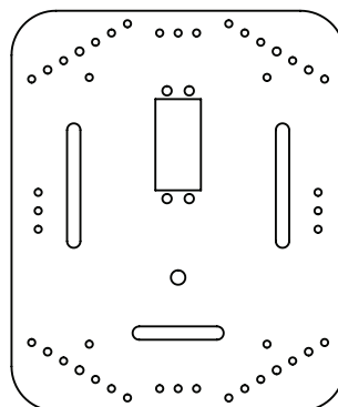
A0 M0306x1 车身上板 Upper Deck
