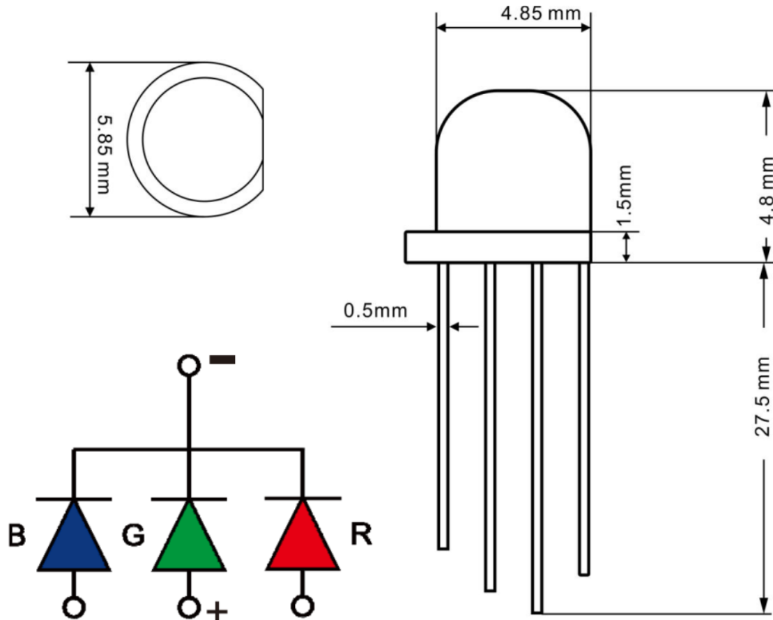
Emitter外型图:
