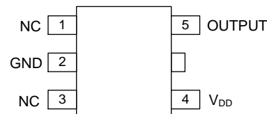
SOT553
