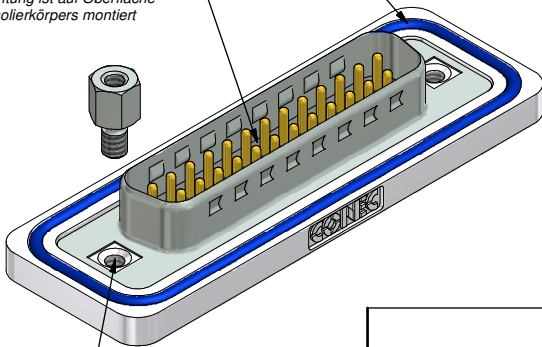
Threaded insert/ Gewindeeinsatz
