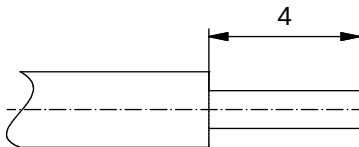
Stripping Dimensions/ Kabelvorbereitung:
