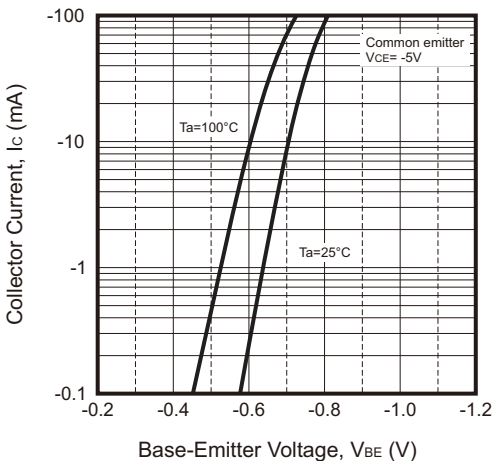
Fig.5 - I_c — V_{BE}
