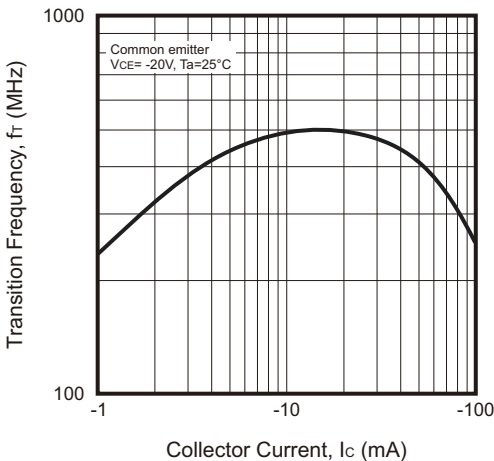
Fig.7 - f_r — I_c
