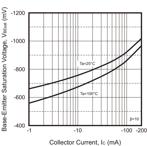
Fig.4 - V_{BEsat} — I_c
