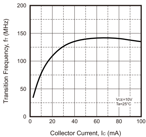
Fig.5 - f_r — I_c
