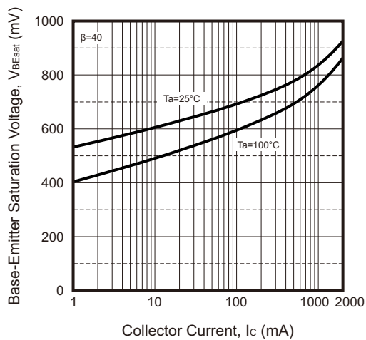
Fig.3 - V_{BEsat} — I_c
