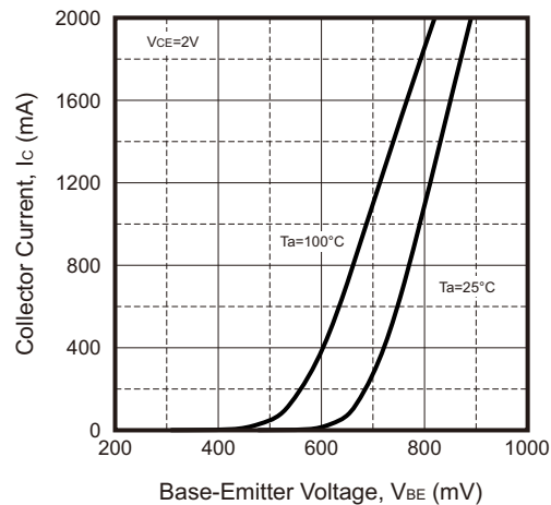
Fig.7 - V_{BE} — I_C
