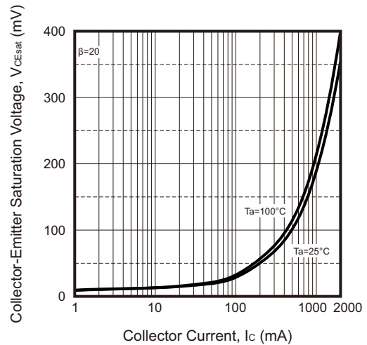
Fig.4 - V_{CEsat} — I_c
