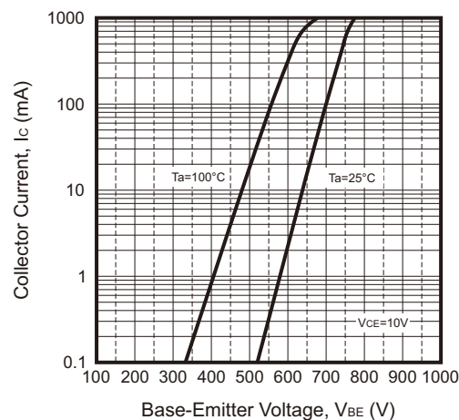
Fig.6 - I_c — V_{BE}
