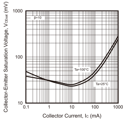
Fig.4 - V_{CEsat} — I_c
