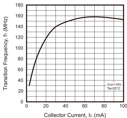
Fig.5 - f_T — I_c
