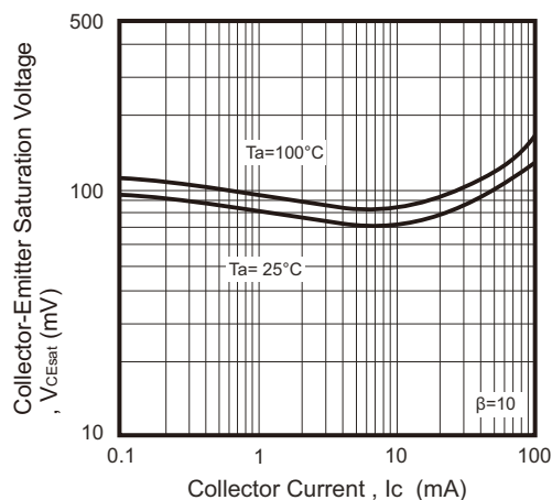
Fig.3 - V_{CEsat} - I_C
