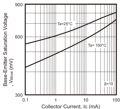
Fig.4 - V_{BEsat} - I_C
