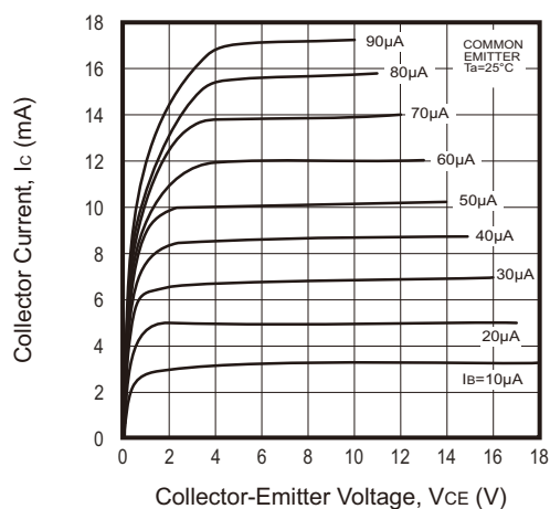
Fig.1 - I_C - V_{CE}
