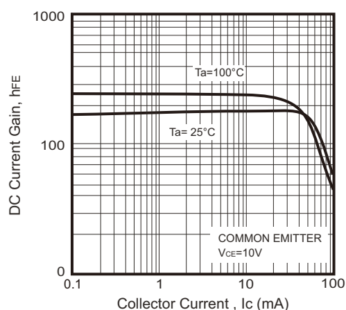
Fig.2 - h_{FE} - I_C
