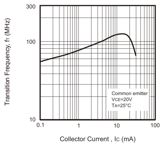
Fig.6 - f_T — I_C
