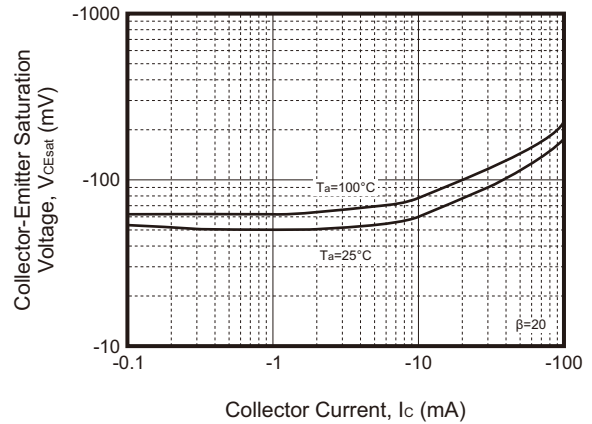
Fig.4 - V_{CEsat} — I_c
