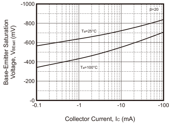
Fig.3 - V_{BEsat} — I_c
