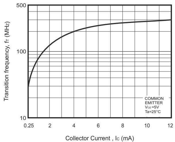
Fig.6 - f_T - I_C
