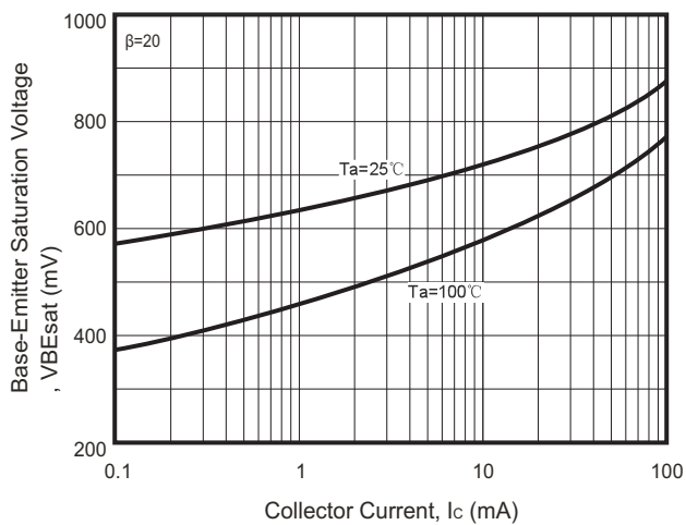
Fig.3 - V_{BEsat} - I_C
