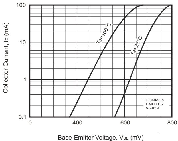
Fig.5 - I_C - V_{BE}
