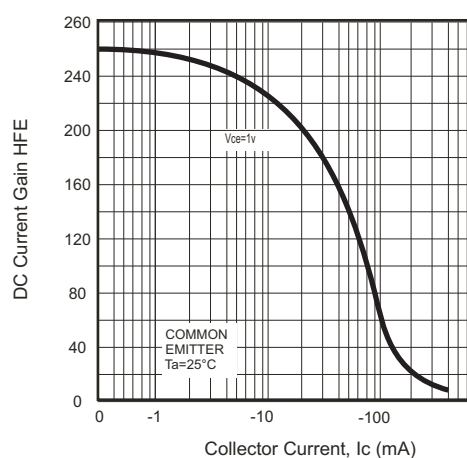
Fig.4 - h_{FE} - I_c
