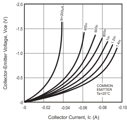
Fig.2 - V_{ce} - I_c
