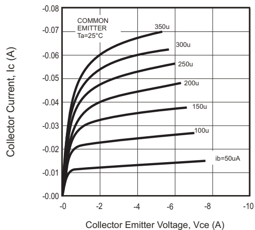
Fig.1 - I_c - V_{ce}
