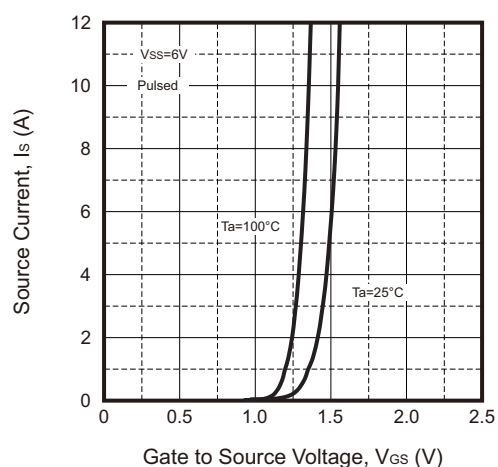
Fig.2 - I_S — V_{GS}
