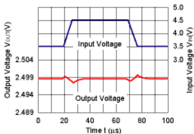
2.5V(VR2)
