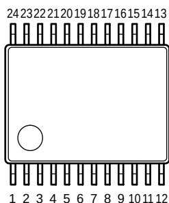
SSOP-24
