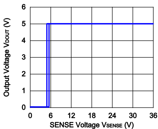
R3150NxxxE ( -V_{DET} = 5.0\text{ V} , +V_{DET} = 5.3\text{ V} )
