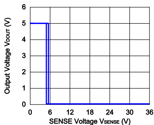
R3150NxxxF ( -V_{DET} = 5.0\text{ V} , +V_{DET} = 5.3\text{ V} )
