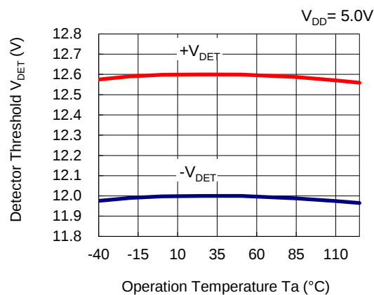
R3121N120E
