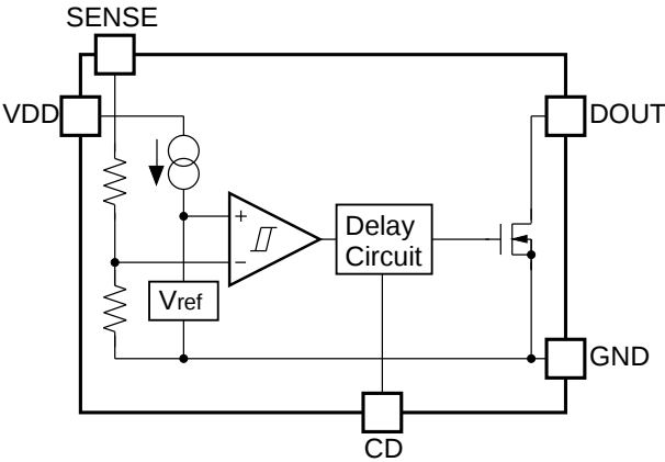
R3121NxxxE
