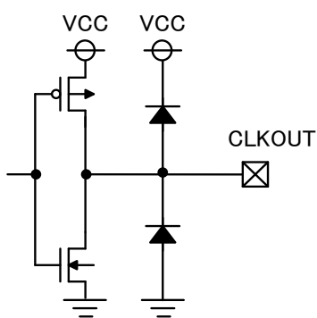
&lt; CLKOUT Pin &gt;
