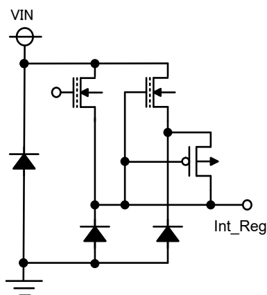
&lt; VIN Pin &gt;
