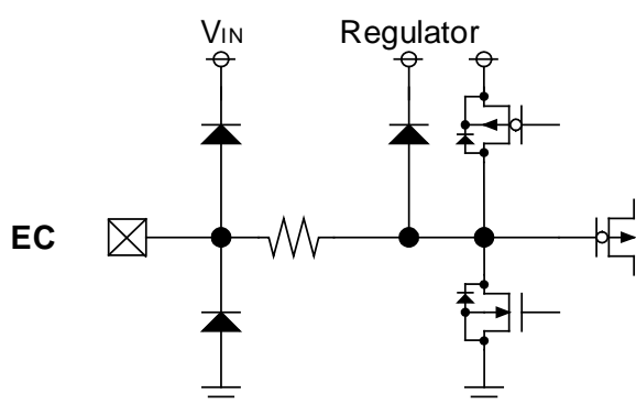
&lt;EC Pin&gt;
