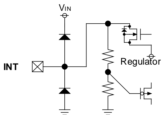
&lt;INT Pin&gt;
