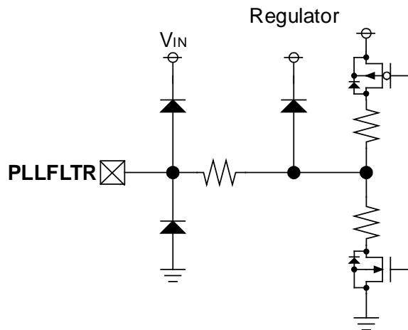
<PLLFLTR Pin>
