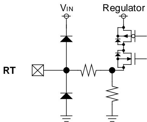
<RT Pin>
