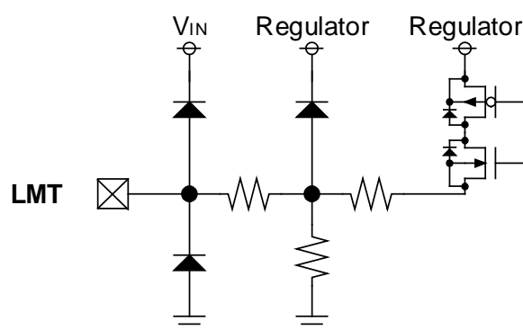
&lt;LMT Pin&gt;
