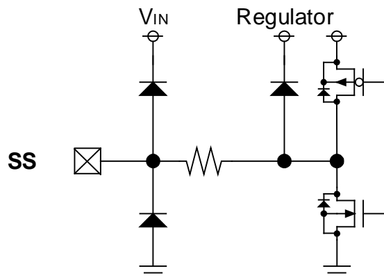
<SS Pin>
