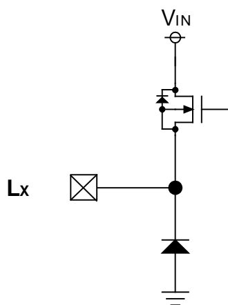
&lt;Lx Pin&gt;
