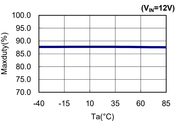
12) Maxduty(ver.A,B Rt=floating)
