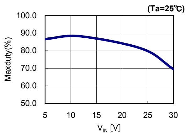
16) Maxduty(ver.C,D)
