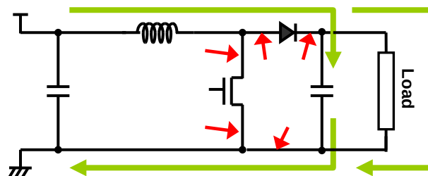
Fig. 4 MOSFET-OFF
