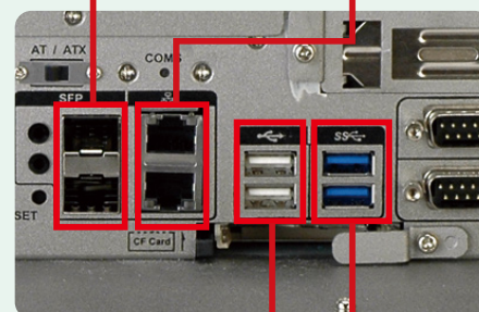
Fiber LAN
