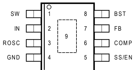
(8 - Pin SOIC - EDP)
